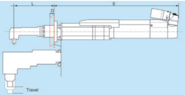
QST - CTV nutrunner
